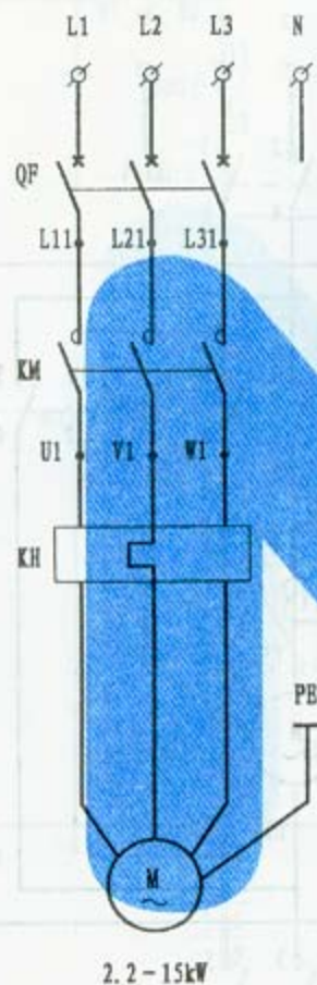
水泵电机
