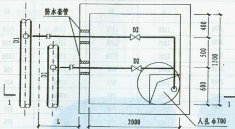
平面图
