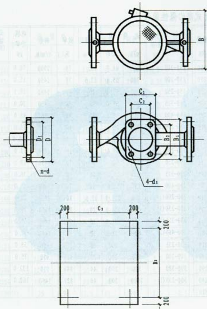
基础平面图
