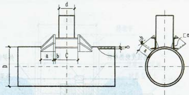
II型加固方案
