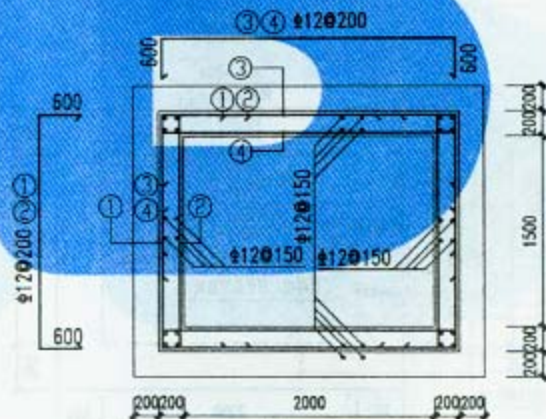
壁板配筋图
