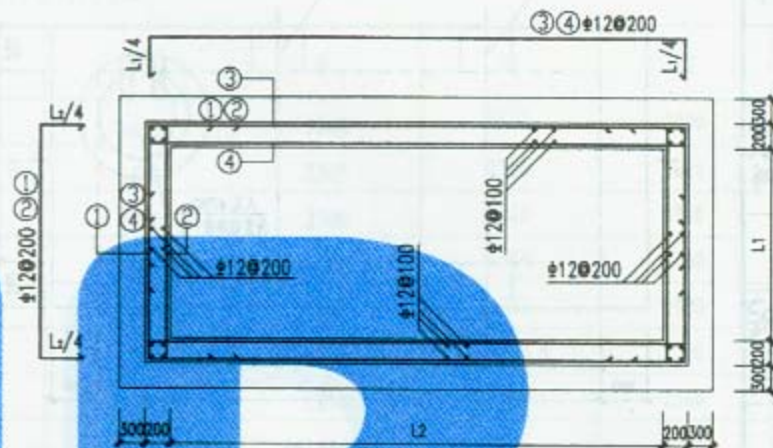
墙板配筋图
