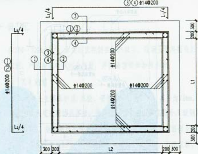
墙板配筋图
