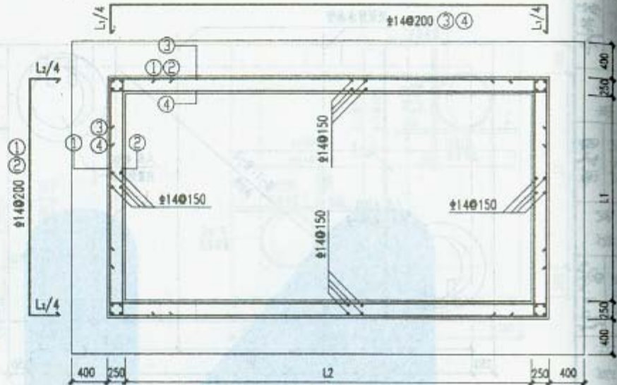
壁板配筋图
