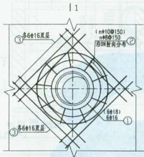
防水套管加固图
