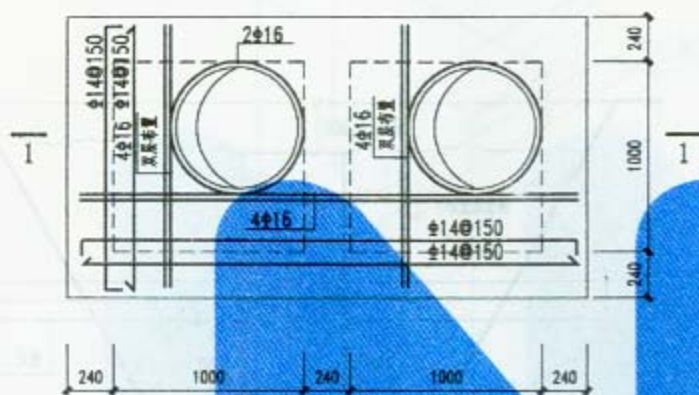
顶板配筋图
