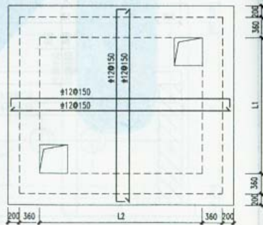
底板配筋图
