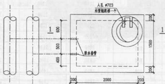
平面图
