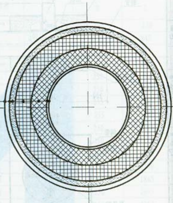
硬质保温结构
